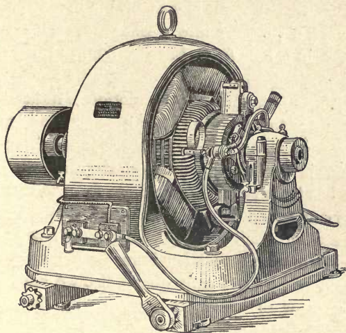
FIG. 7.—Dynamo.
